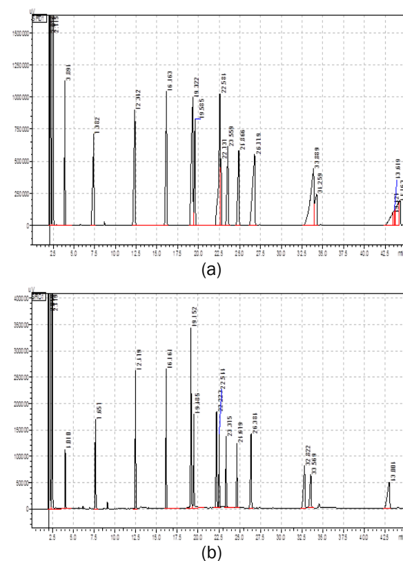
Gambar 2. Kromatogram senyawa FAME. (a) analisis awal; (b) ulangan 1
