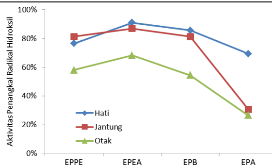
Gambar 2. Grafik aktivitas penangkal radikal hidroksil dari dari ekstrak partisi petroleum eter (EPPE), ekstrak partisi etil asetat (EPEA), ekstrak partisi n -butanol (EPB) dan ekstrak partisi akuades (EPA).
