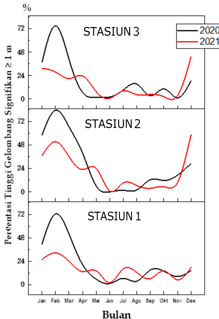
Gambar 6. Proporsi Bulanan Tinggi Gelombang Signifikan Dengan Besaran Lebih Dari 1 Meter Pada Lokasi Penelitian.
