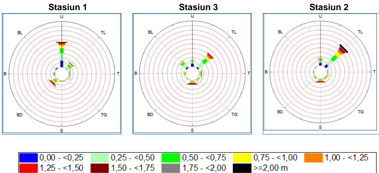
Gambar 2. Mawar Gelombang Yang Menampilkan Tinggi Gelombang Signifikan Pada Ketiga Stasiun di Lokasi Penelitian sepanjang 2020 dan 2021.
