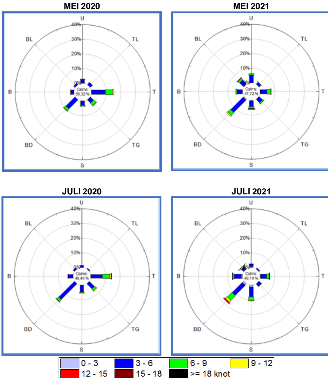
Gambar 8. Arah dan Kecepatan Angin Pada Bulan Mei dan Juli Tahun 2020 dan 2021 Yang Terukur di Stasiun Cuaca Naha.
