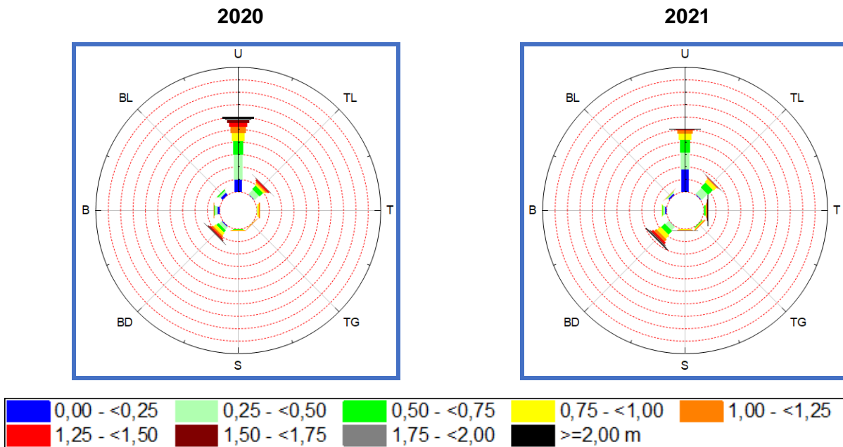
Gambar 3. Mawar Gelombang Yang Menampilkan Tinggi Gelombang Signifikan Pada Stasiun 1 di Lokasi Penelitian.
