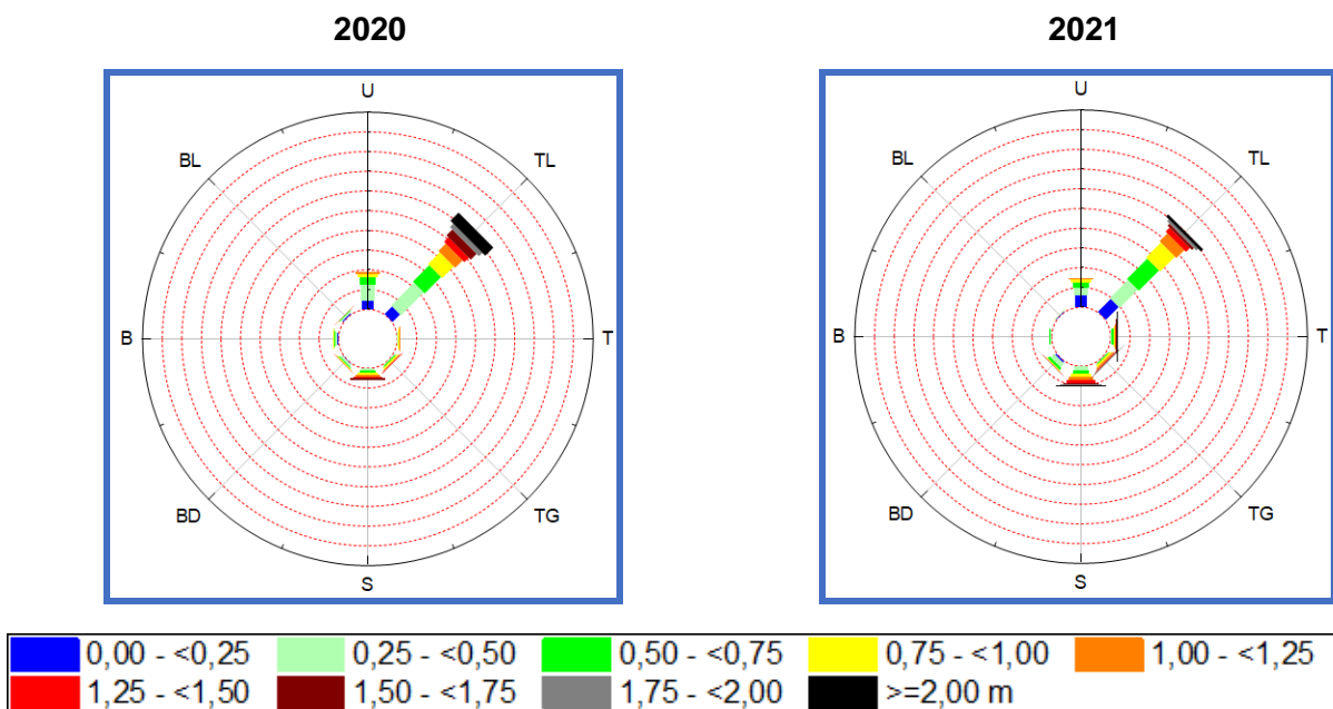
Gambar 4. Mawar Gelombang Yang Menampilkan Tinggi Gelombang Signifikan Pada Stasiun 2 di Lokasi Penelitian.
