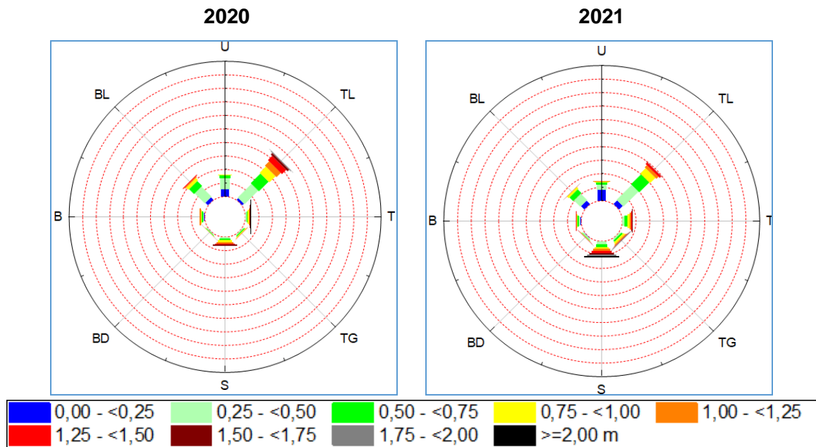
Gambar 5. Mawar Gelombang Yang Menampilkan Tinggi Gelombang Signifikan Pada Stasiun 3 di Lokasi Penelitian.
