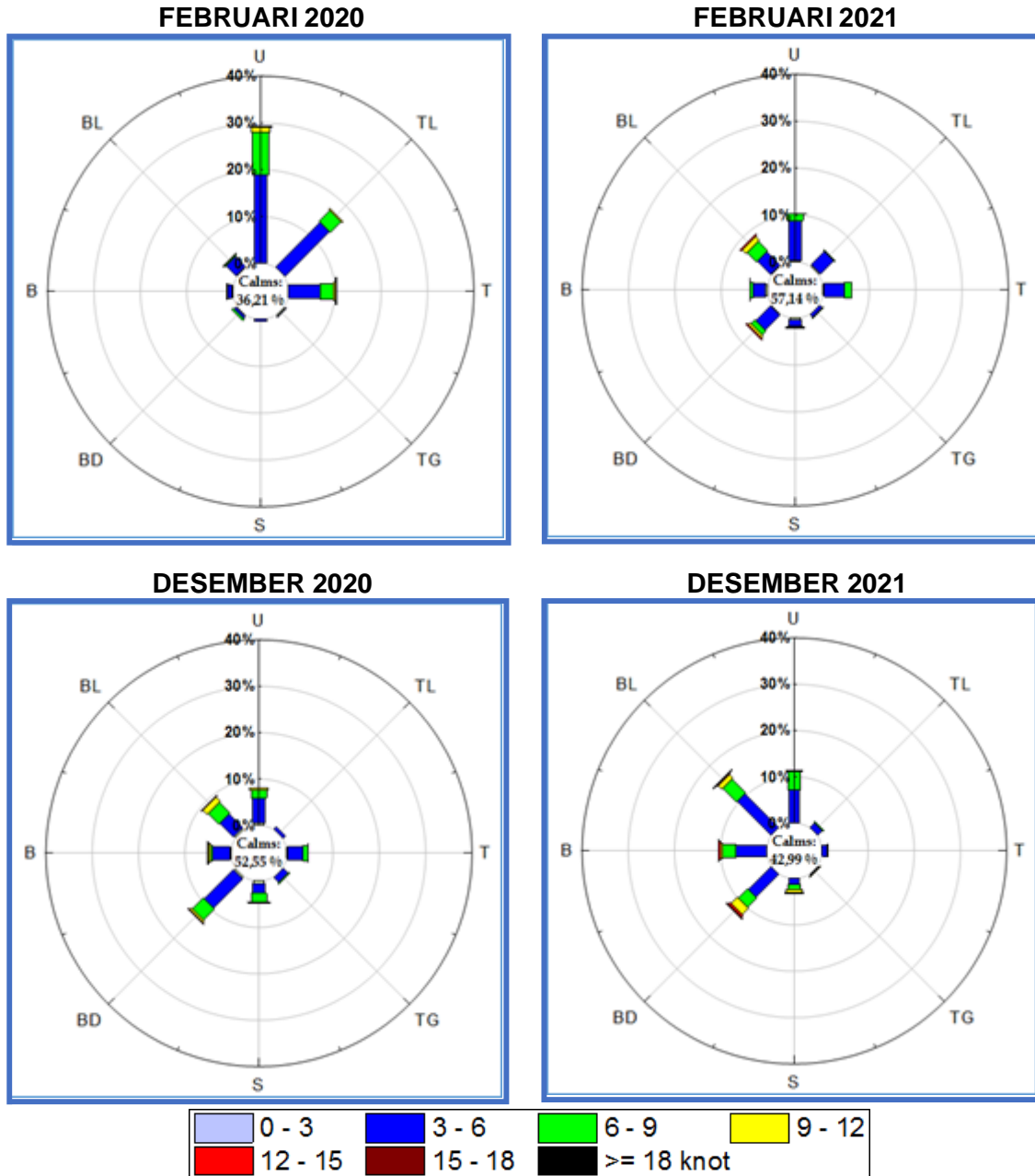
Gambar 7. Arah dan Kecepatan Angin Pada Bulan Februari dan Desember Tahun 2020 dan 2021 Yang Terukur di Stasiun Cuaca Naha.
