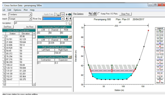
Gambar 11 : Memasukan Data Potongan Melintang
