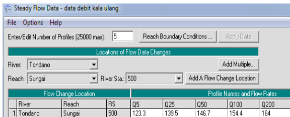
Gambar 10 : Memasukan debit kala ulang tertentu
