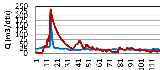
Gambar 4 : Grafik Perbandingan Debit Terukur dan Debit Hitungan
