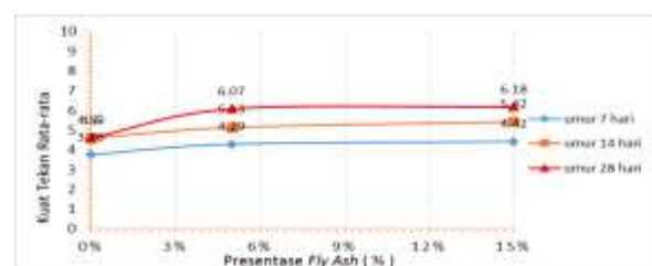
Gambar 7. Hubungan antara kuat tekan mortar rata-rata terhadap persentase abu terbang ( fly ash ).
