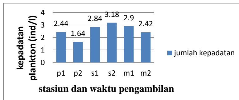
Gambar 02. Kepadatan Plankton
