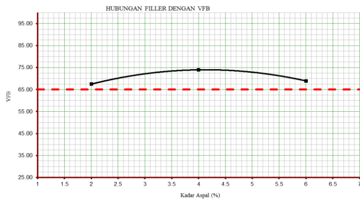
Gambar 13. Nilai VFB Dengan Bahan Tambah
