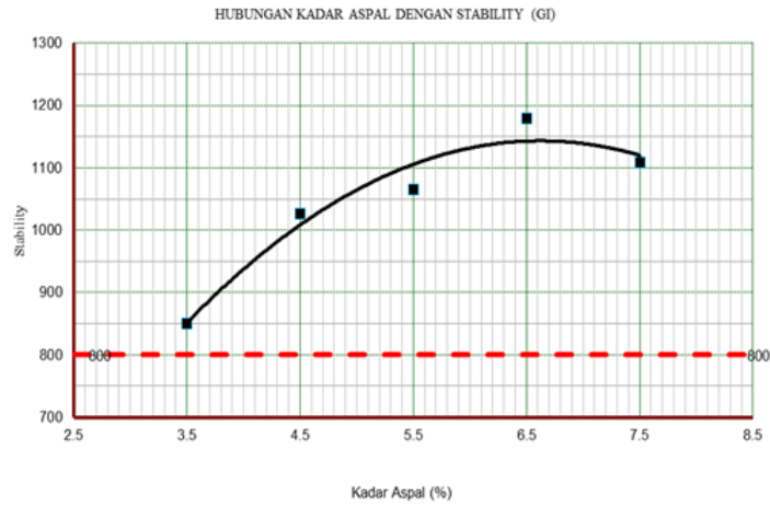
Gambar 5. Stabilitas Tanpa Bahan Bakar
