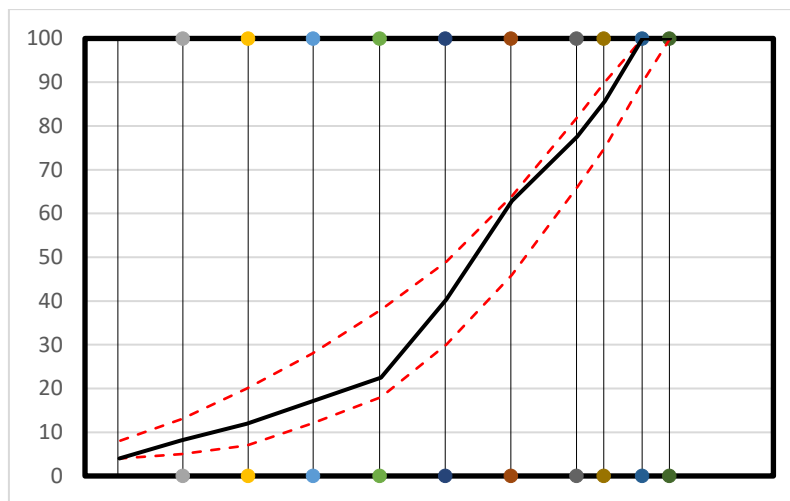
Gambar 3. Grafik Kombinasi Agregat
