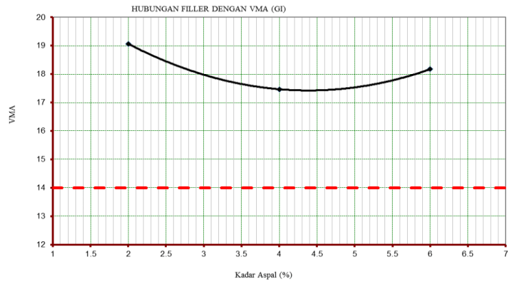
Gambar 12. Nilai VMA Dengan Bahan Tambah
