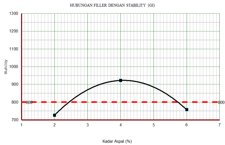
Gambar 10. Stabilitas dengan Bahan Tambah
