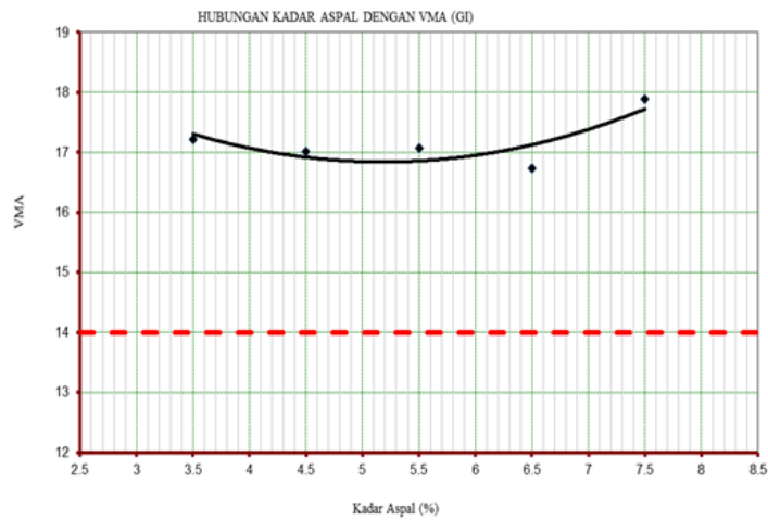
Gambar 7. Nilai VMA Tanpa Bahan Tambah
