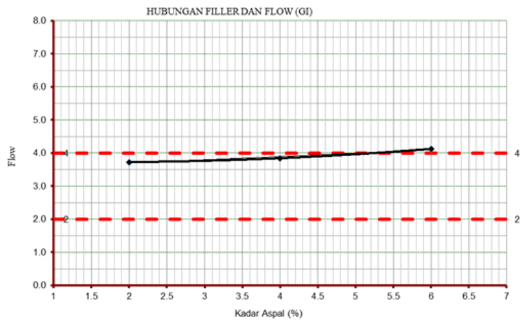
Gambar 9. Nilai Flow Dengan Bahan Tambah
