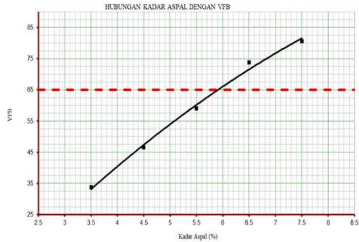
Gambar 8. Nilai VFB Tanpa Bahan Tambah
