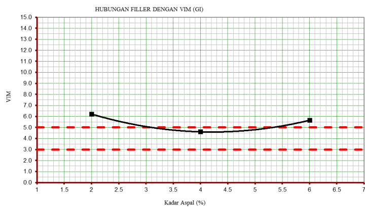
Gambar 11. Nilai VIM Dengan Bahan Tambah
