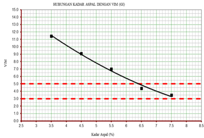
Gambar 6. Nilai VIM Tanpa Bahan Tambah
