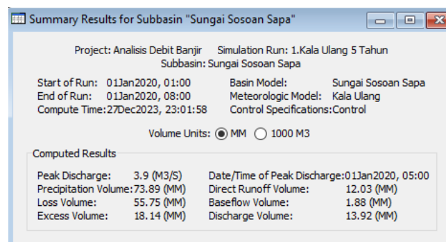
Gambar 6. Summary Result Kala Ulang 5 Tahun
