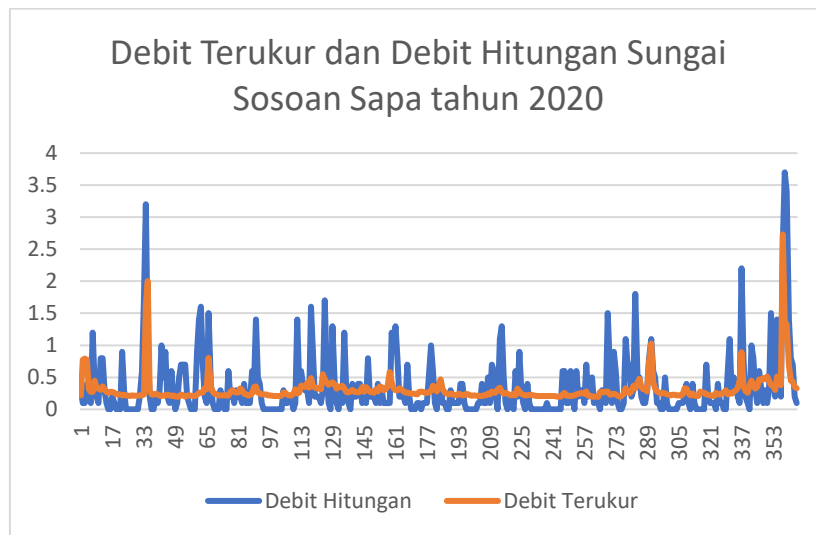
Gambar 5. Grafik Debit Hasil Perhitungan dan Debit Terukur
