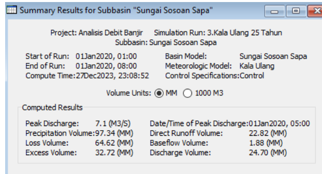
Gambar 8. Summary Result Kala Ulang 25 Tahun
