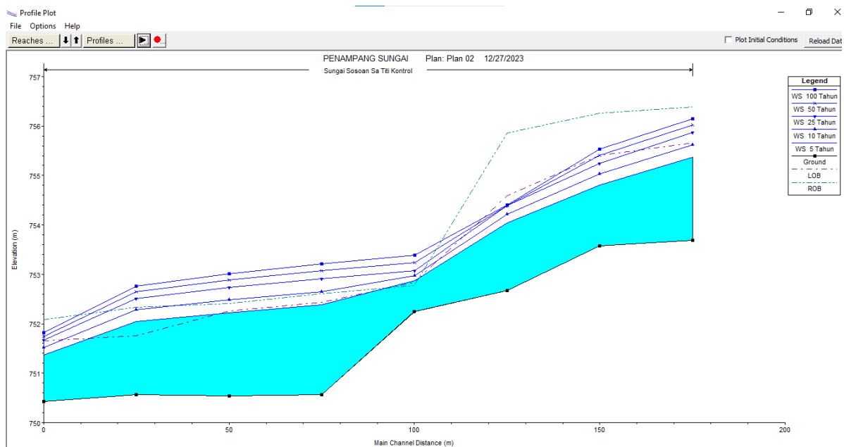
Gambar 14. Rangkuman Elevasi Tinggi Muka Air Profil Memanjang Sungai Sosoan Sapa di Titik Kontrol
