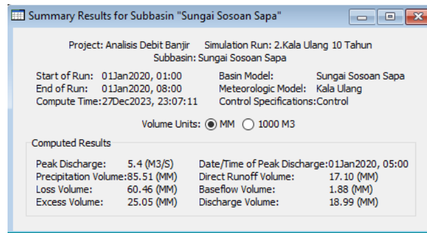
Gambar 7. Summary Result Kala Ulang 10 Tahun
