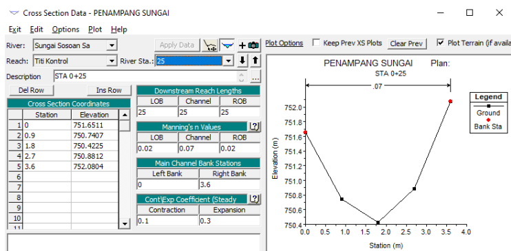
Gambar 11. Data Penampang Melintang Sungai STA 0+25
