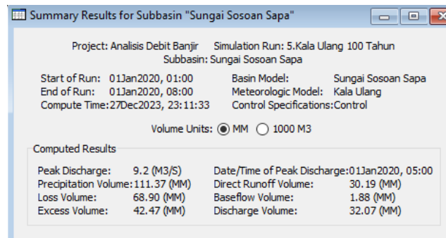
Gambar 10. Summary Result Kala Ulang 100 Tahun
