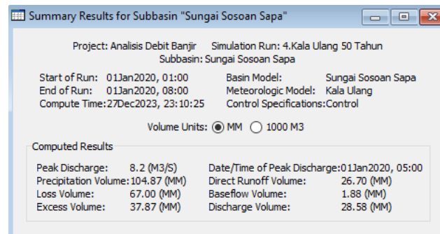
Gambar 9. Summary Result Kala Ulang 50 Tahun
